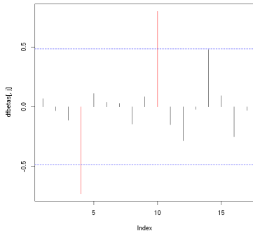
DFBETAS - Experiencia
