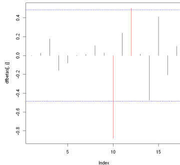
DFBETAS - Escolaridade
